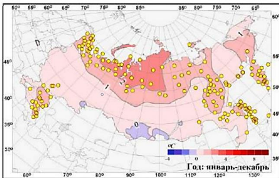
Аномалии средней годовой и сезонных температур приземного воздуха на территории РФ в 2022 г. (отклонения от средних за 1991-2020 гг.) с указанием локализации 95%-х экстремумов (желтые кружки)
