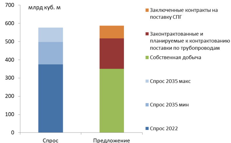
Баланс газа в Китае на 2035 г.
